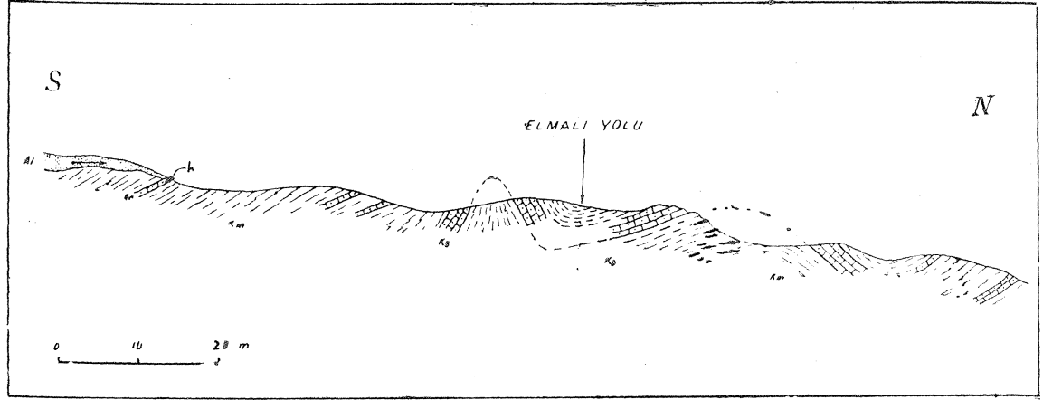
Şekil 2 - Biğer köjii cıran^ Töprakpınar deresi kesiii
