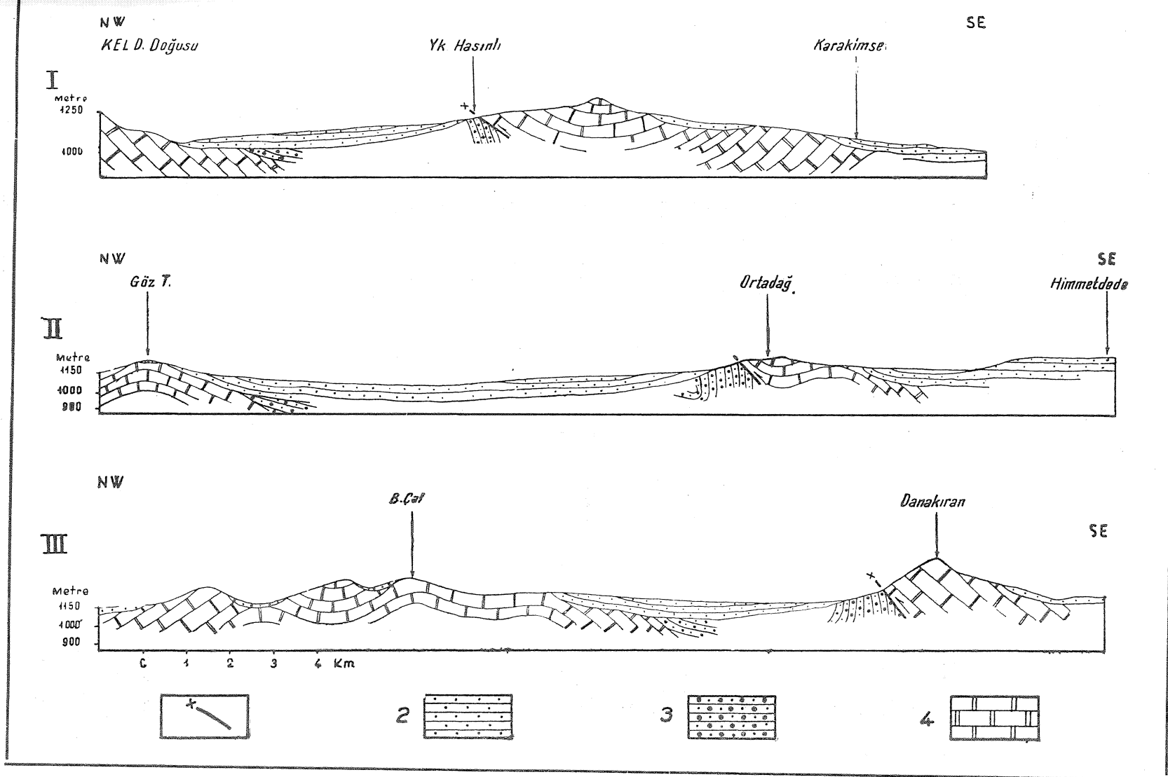
Şekil 1 - Himmetdede civarının jeolojik kesitleri
